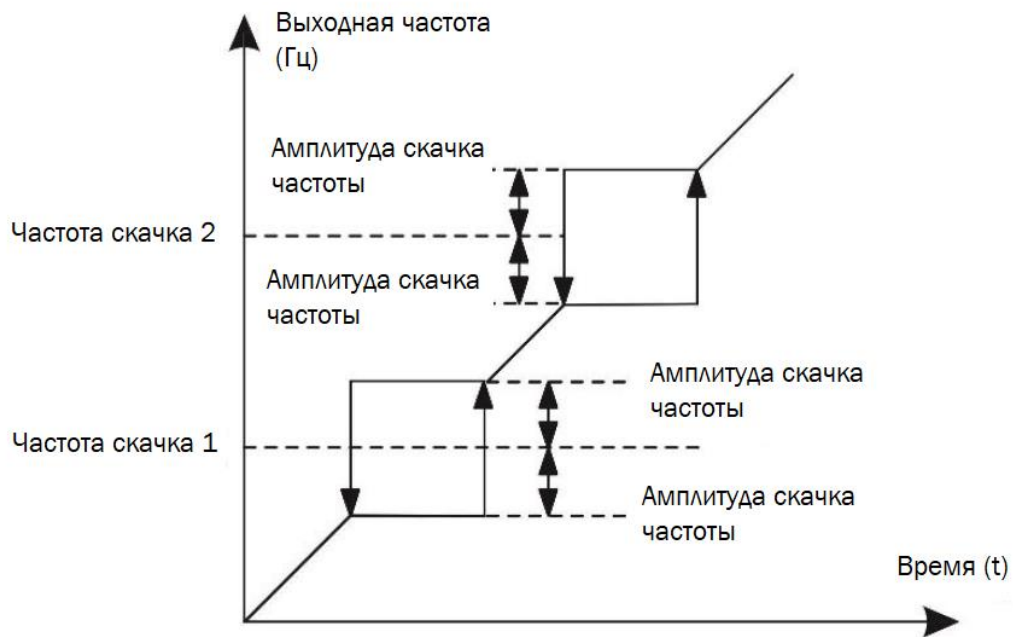
Рисунок 6-13 - Принцип работы скачка частоты
