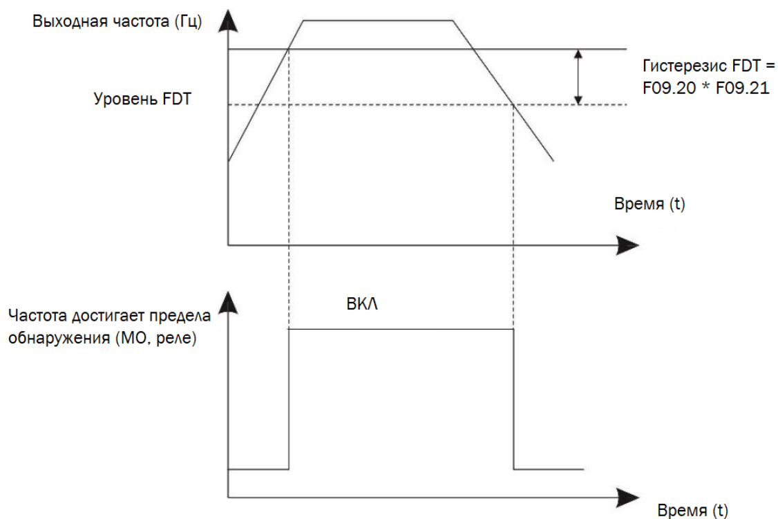
Рисунок 6-15 – Функция FDT
