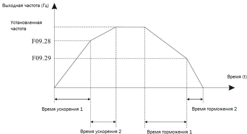
Рисунок 6-16 – Переключение между t ускорения 1 и 2 / торможения 1 и 2
