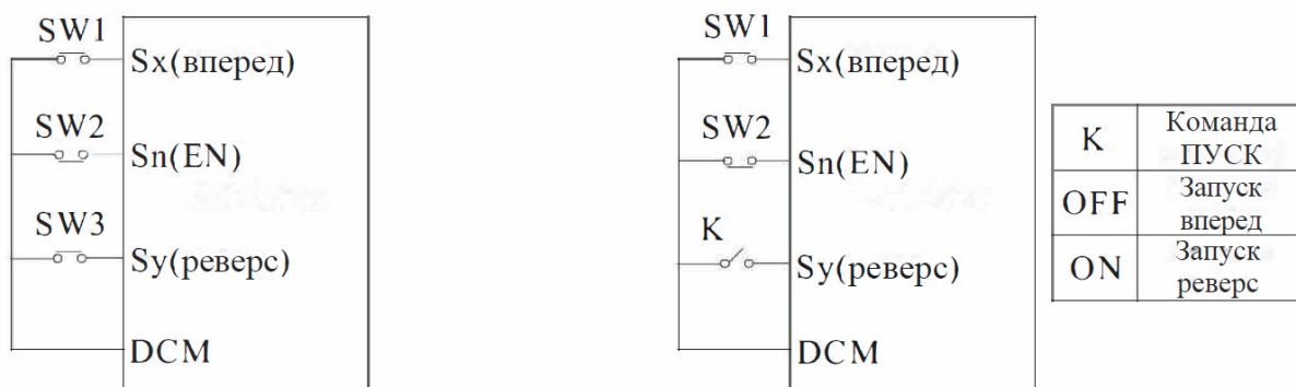
Рисунок 6-10 – Настройка 3-х проводного управления 1 и 2
